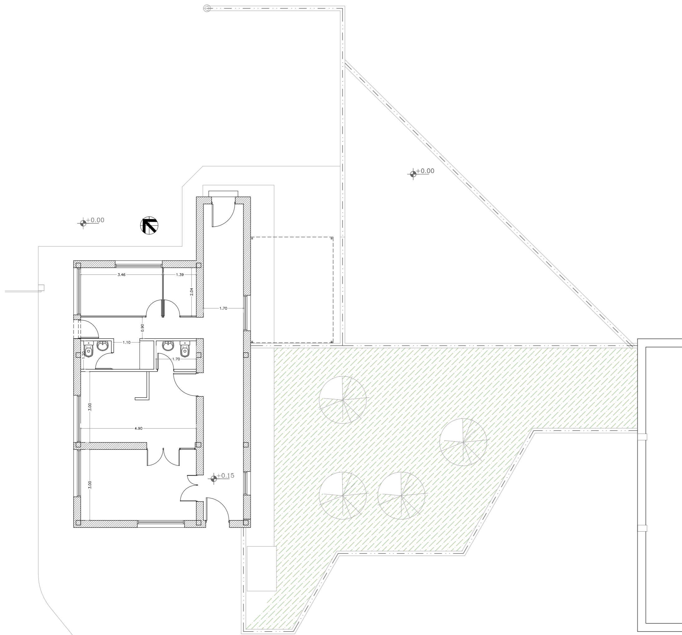
PLANTA AREA MOV. DE SUELOS ESC. 1:100
