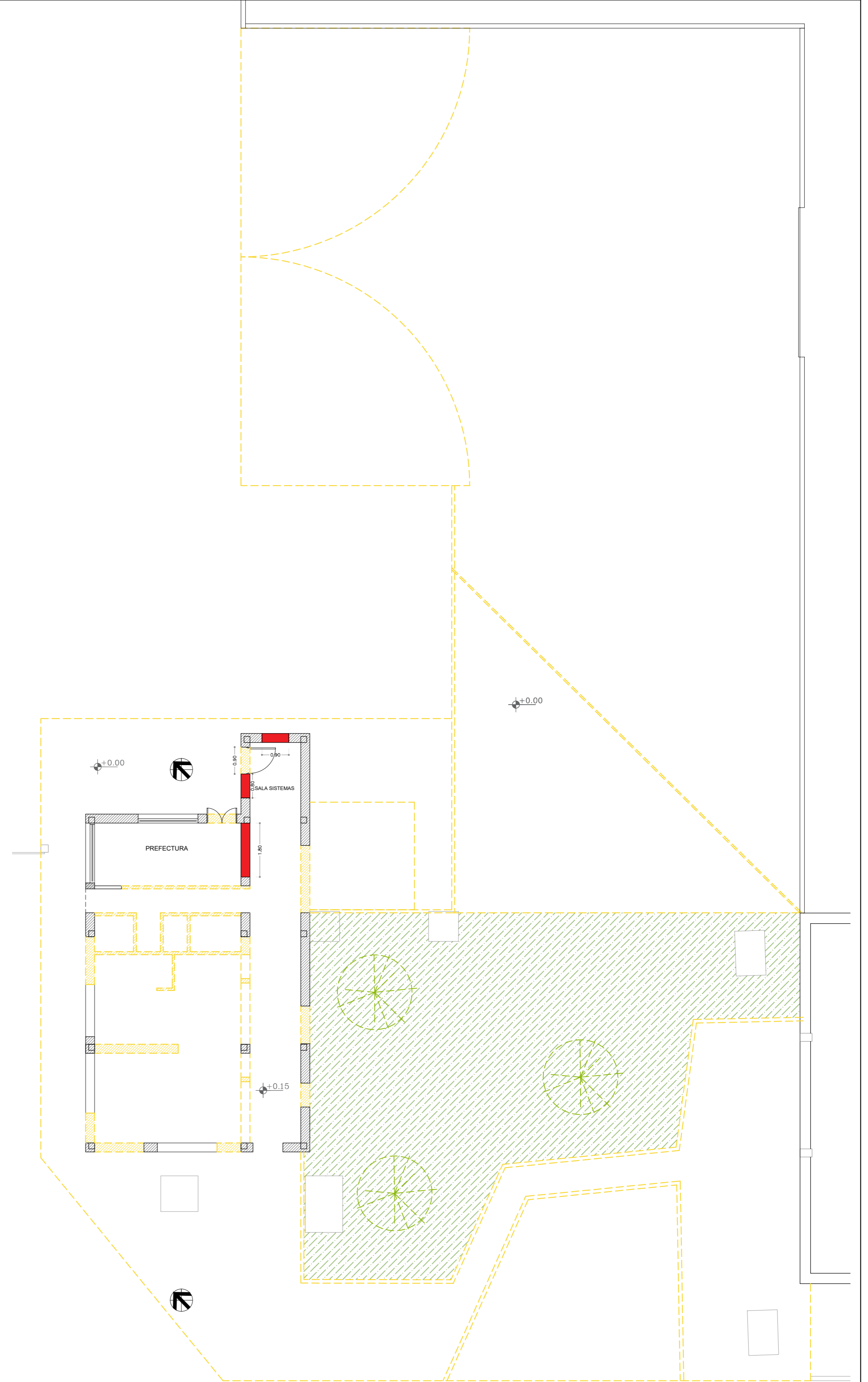
PLANTA DEMOLICIONES ESC. 1:100
